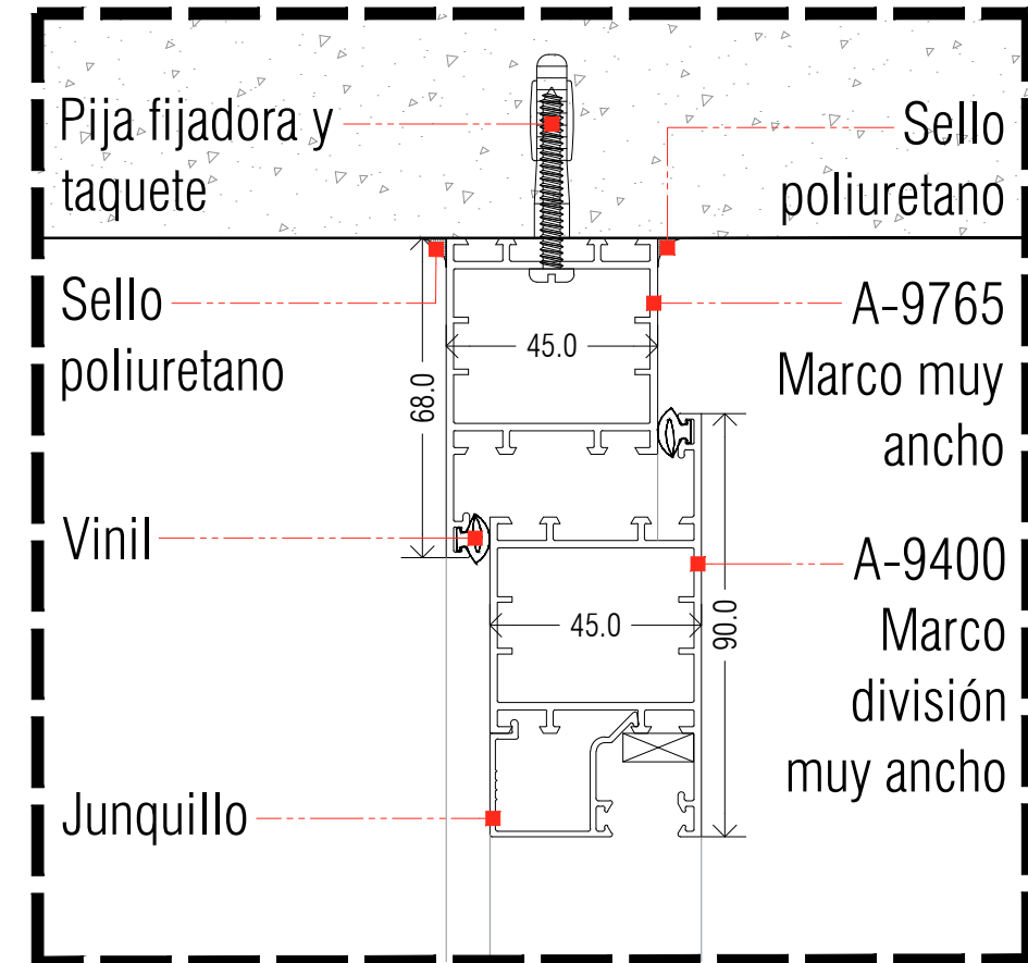
Corte B
