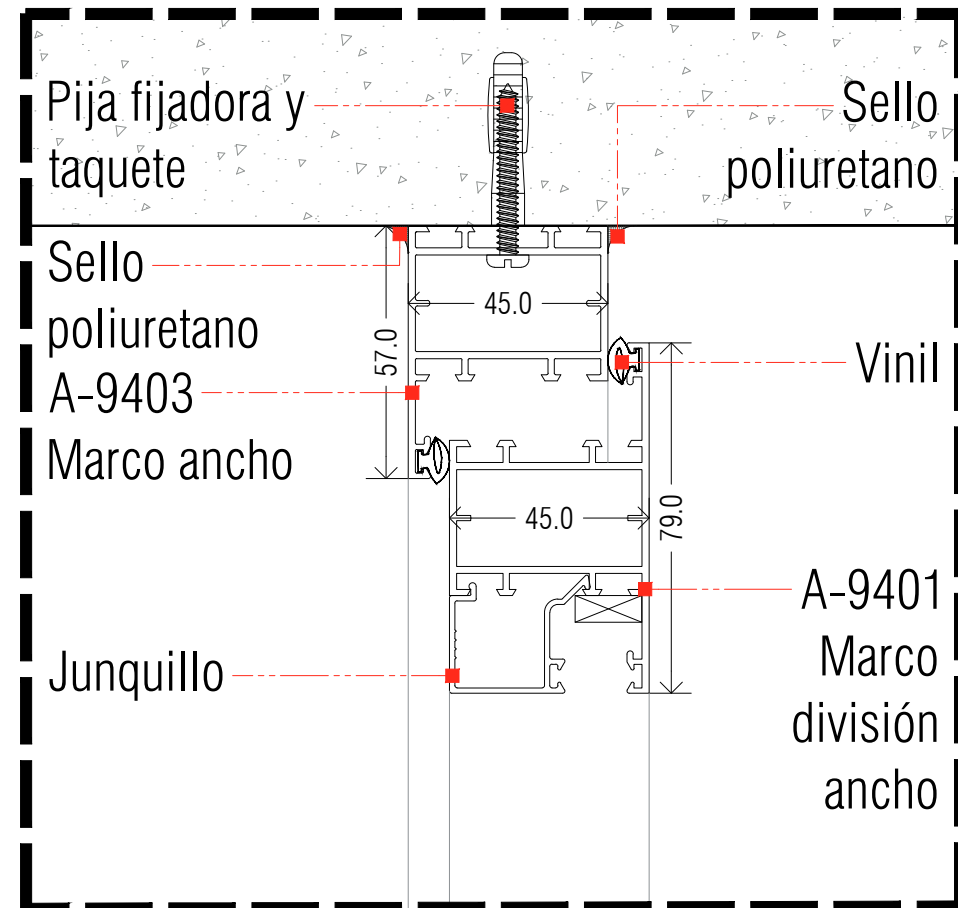
Corte B
