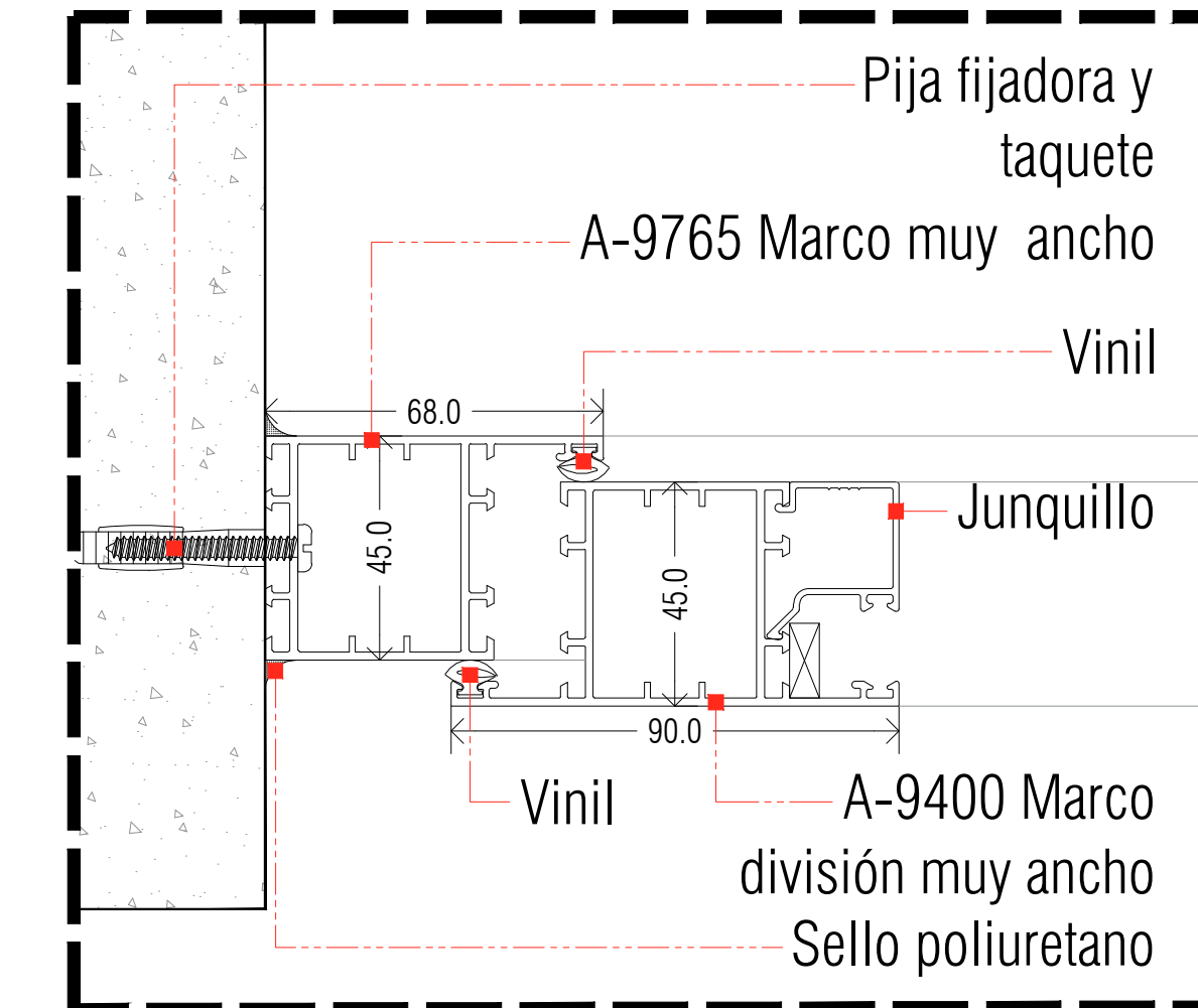
Corte A
