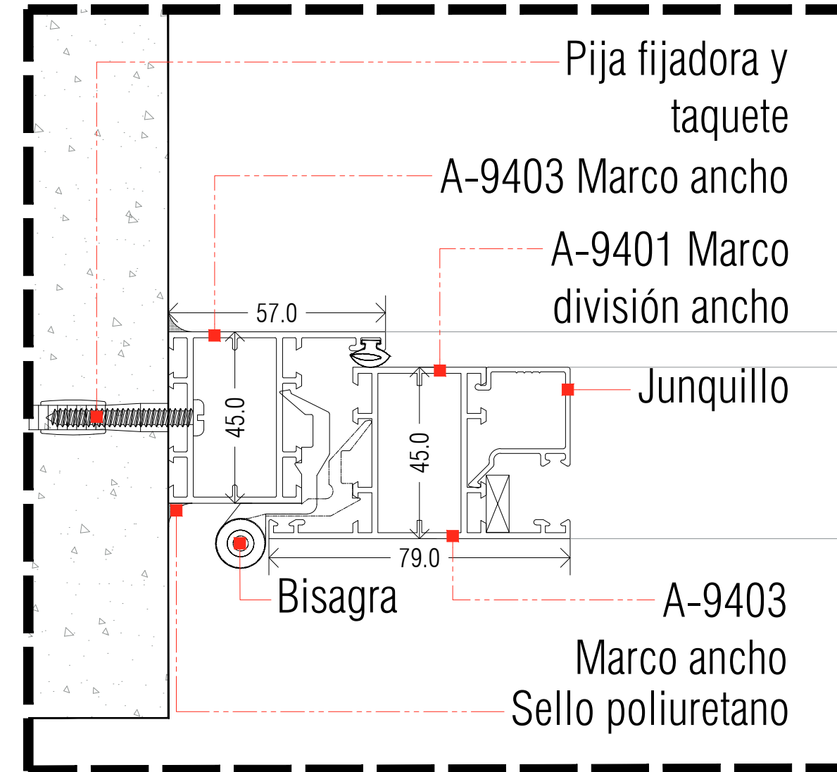
Corte A
