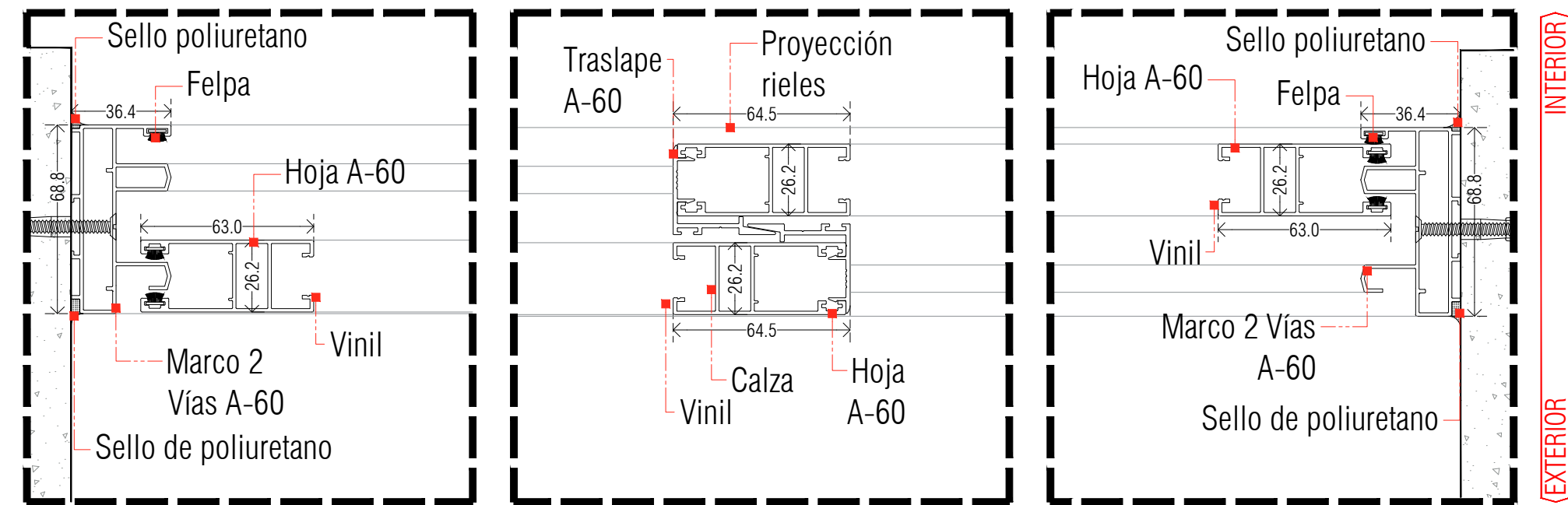
Corte A
