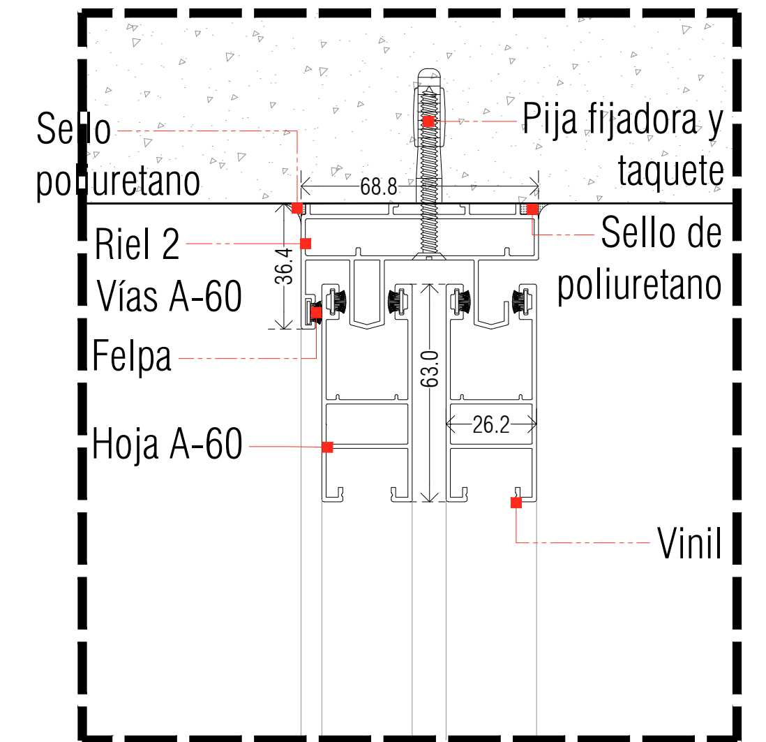
Corte B
